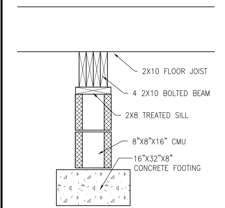
PIER DETAIL SCALE 1"=1'-0" F1
